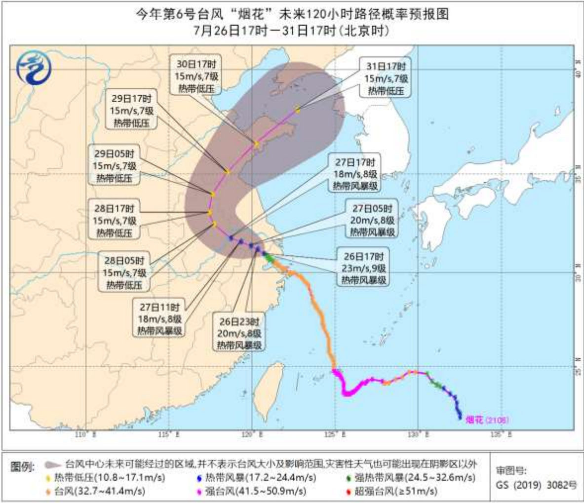
图1 第6号台风“烟花”移动路径预报图
